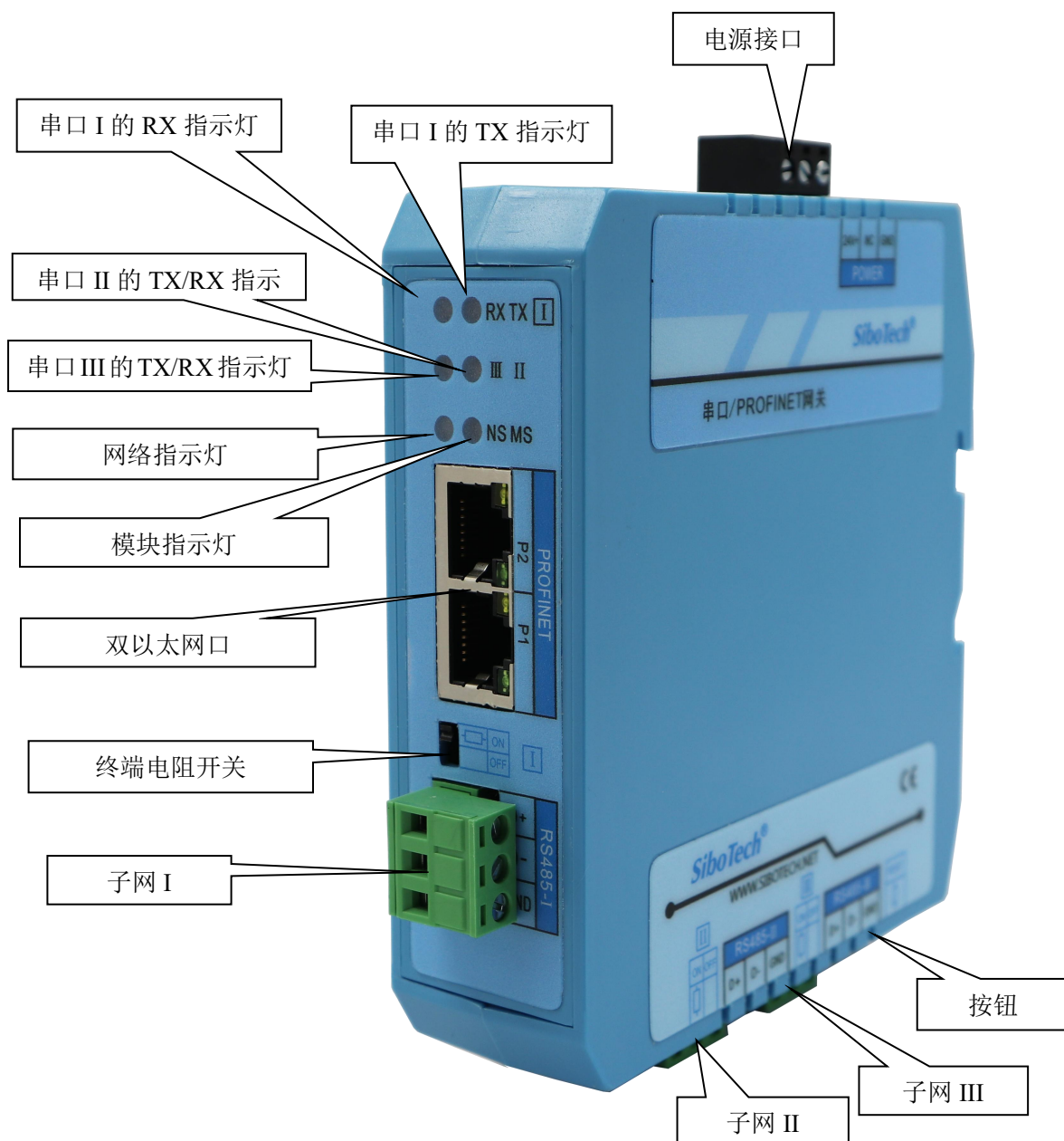
图 1 产品外观
