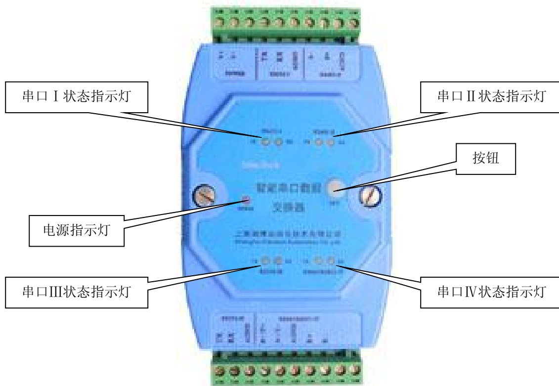
图 1 产品外观
